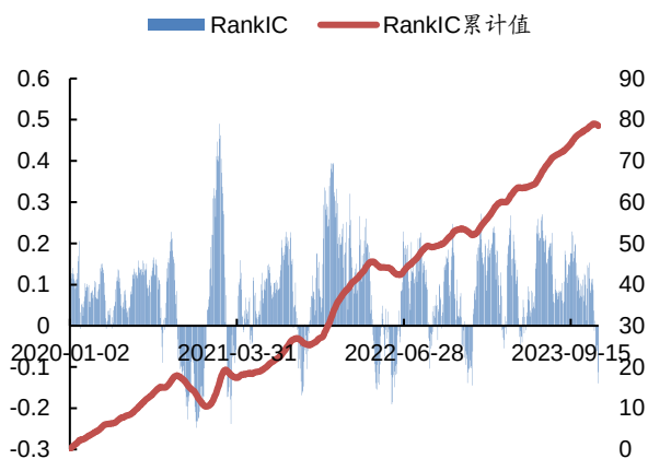
图 19: 精选大小单因子组合RankIC (创业板)
