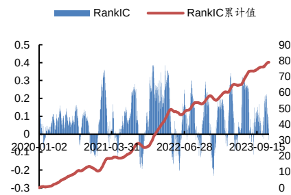
图 2：精选大小单因子组合 RankIC
