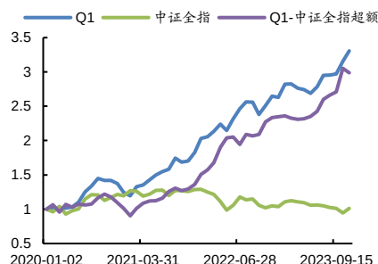
图 1：精选大小单因子组合表现
